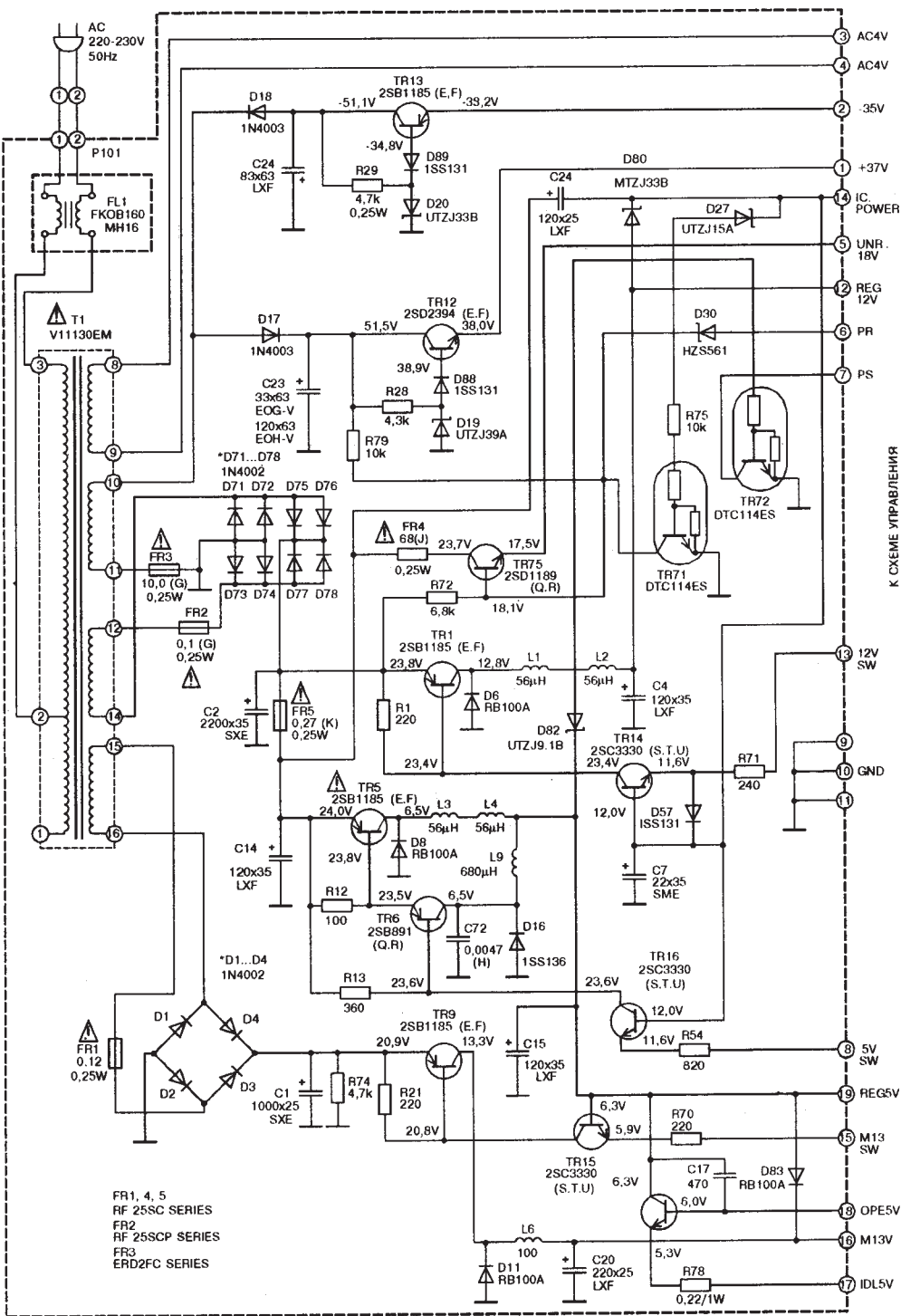
Принципиальная схема трансформаторного блока источника питания видеомагнитофонов VS-G44EOH-V/G45EOG-V
